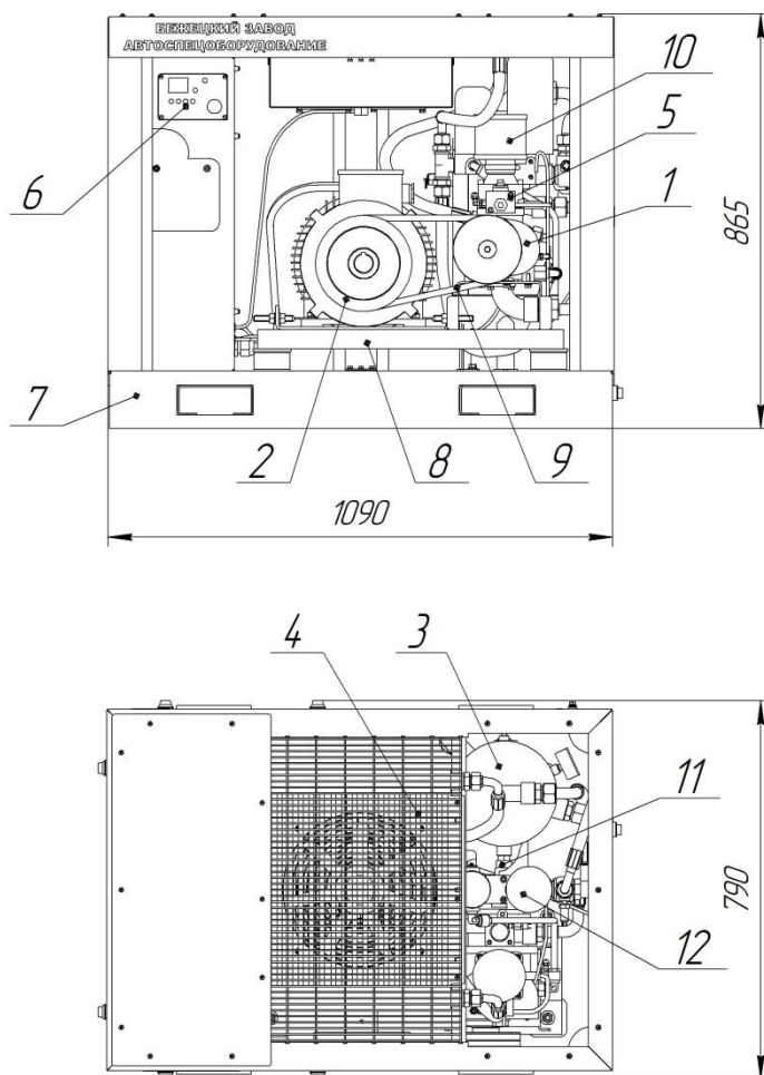
Рисунок 2. Агрегат компресорний
